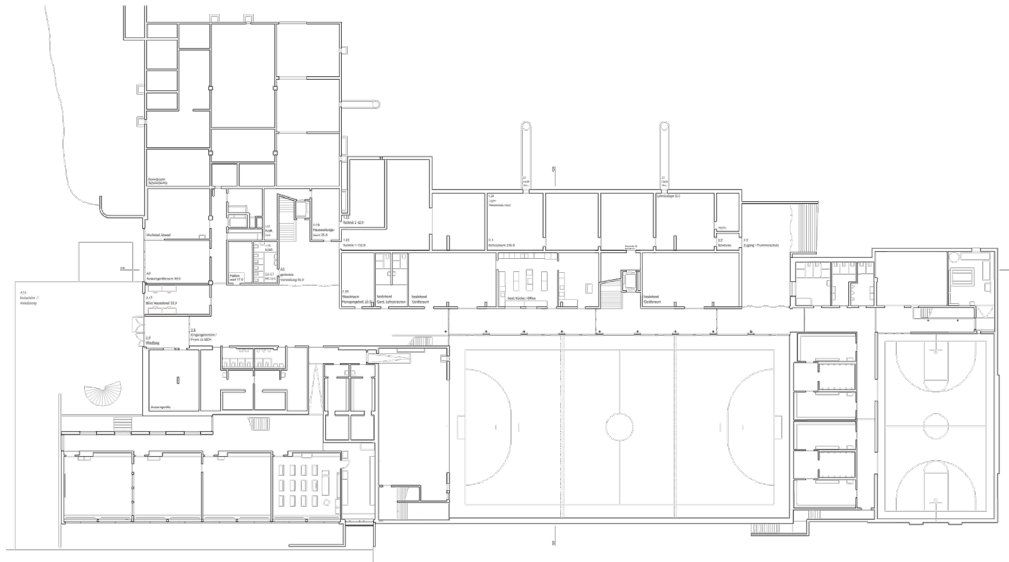
Grundriss Untergeschoss
