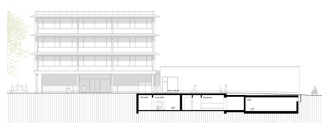
Ansicht West
