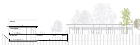
Querschnitt Annex und Ansicht Ost Aulagebäude
