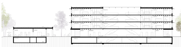
Längsschnitt
