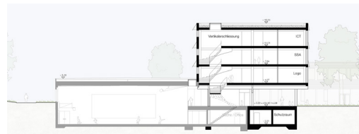
Querschnitt
